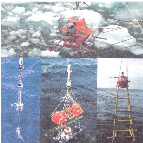
【上】南極海における海底基準局投入 【左】モーター式リリーストランスポンダ 【中】精密測距装置/海底基準局 【右】チタン製耐圧球 650mm
